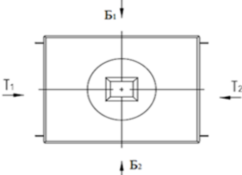
Схема обозначения сторон ККС-2,5-10 ССД-Пайп (вид сверху)
