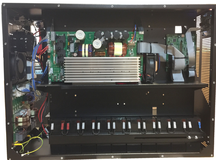
Рисунок 5 – Расположение батарей 7/9 Ач Trio TT
