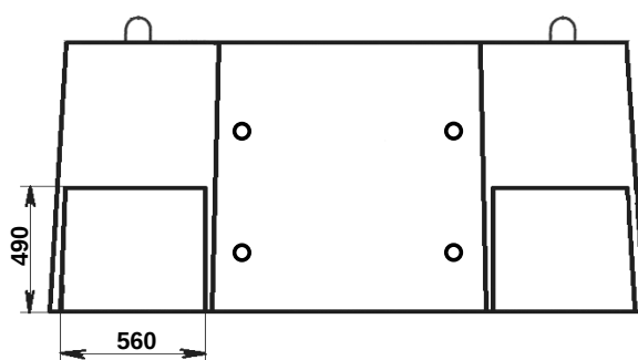
Рис. 7. Размеры ниш на примере верхнего элемента колодца «ККСр-4-80». На нижнем элементе ниши такого же размера.
