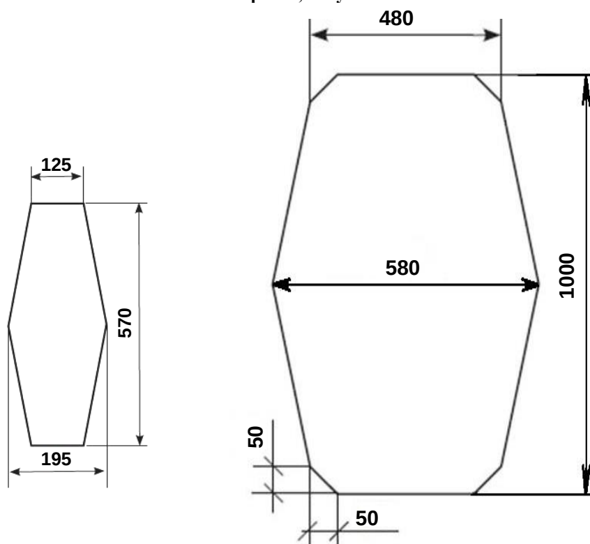
Рис. 2.1. Форма участка с тонкой неармированной стенкой на торцевой стене колодца «ККСр-4-80»: 1 – технологическое отверстие; 2 – участок с тонкой стенкой.
