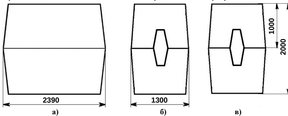
Рис. 5. Габаритные размеры колодца «ККСр-4-80»:
