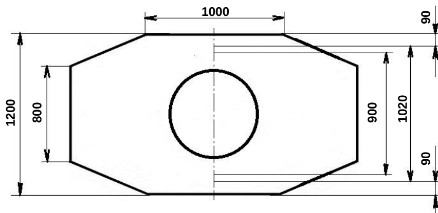
Рис. 6. Размеры перекрытия колодца «ККСр-4-80» с указанием диаметров опорных колец: 900 мм – кольца типа КО; 1020 мм – кольца КО-ЧП и КО-Ч.
