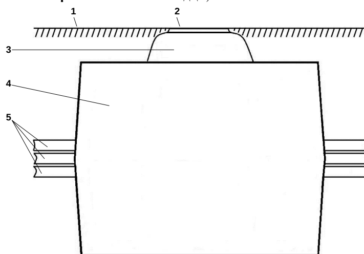
Рис. 2. Колодец «ККСр-4-80» как подземное сооружение: 1 – уровень земли или асфальта; 2 – чугунный люк тяжелого типа; 3 – горловина в бетонной обмазке; 4 – корпус колодца в сборе; 5 – вводимые каналы, 12 труб.
