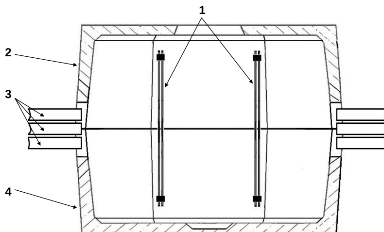
Рис. 11. Ввод труб в колодец «ККСр-4-80»: 1 – кронштейны ККП-130; 2 - торцевая стена верхнего элемента колодца; 3 – ввод хризотилцементных труб в проёмы в торцевых стенах элементов колодца; 4 – торцевая стена нижнего элемента колодца.
