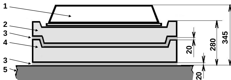
Рис. 14. Высота горловины с парой колец «КО-ЧП» и «КО-Ч»: 1 – люк чугунный типа «Т»; 2 – кольцо «КО-Ч»; 3 – слой бетона со щебнем; 4 – кольцо «КО-ЧП»; 5 – перекрытие колодца «ККСр-4-80».
