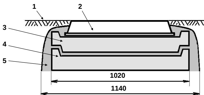
Рис. 15. Диаметры колец и обмазанной бетоном горловины при использовании пары «КО-ЧП» и «КО-Ч»: 1 – уровень земли на газоне, асфальта на тротуаре; 2 – люк лёгкого типа; 3 – кольцо «КО-Ч»; 4 – кольцо «КО-ЧП»; 5 – обмазка горловины бетоном со щебнем.
