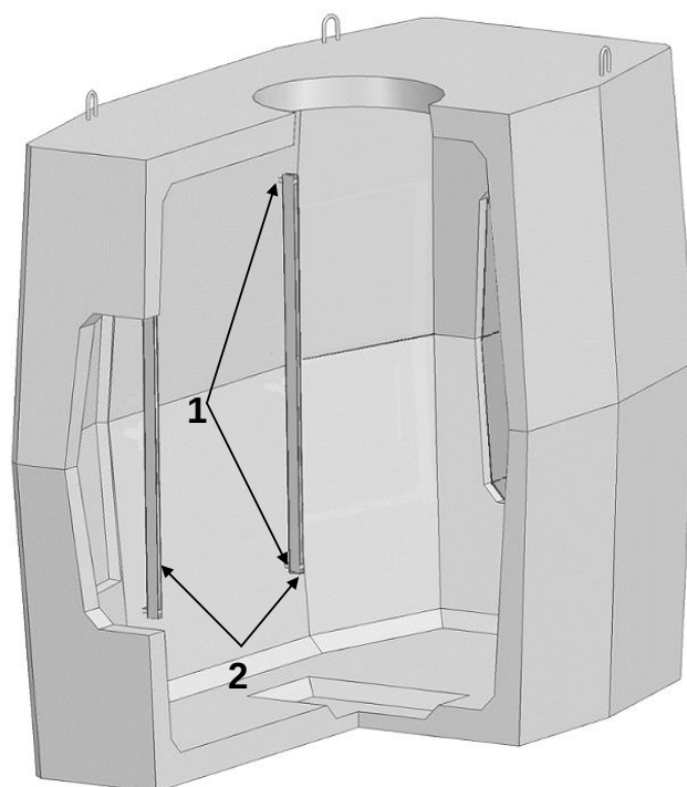
Рис. 3.1. Кронштейны «ККП-130» на боковой стене колодца «ККСр-4-80»: 1 – кронштейны; 2 – ёрши с резьбой.
