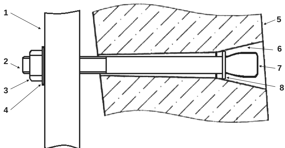
Рис. 3.2. Крепление кронштейна типа ККП с помощью ёршей с резьбой: 1 – кронштейн ККП; 2 – ёрш, конец с резьбой М12; 3 – гайка М12; 4 – шайба; 5 – боковая стена колодца; 6 – отверстие для ёрша; 7 – ёрш, расплющенный конец; 8 – шайба.
