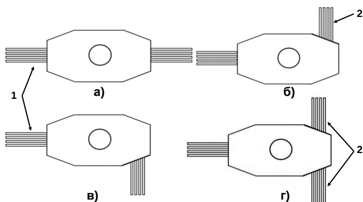
Рис. 3. Классические примеры использования колодца «ККСр-4-80»*: 1 – вводимые каналы; 2 – ответвляющиеся каналы; а - проходной колодец; б, в – угловые колодцы; г - разветвительный колодец.
