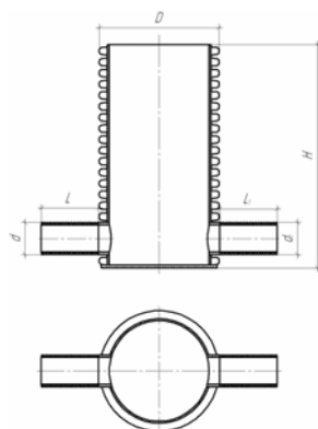
Рисунок Б.12 – Полиэтиленовый сварной безлотковый колодец
