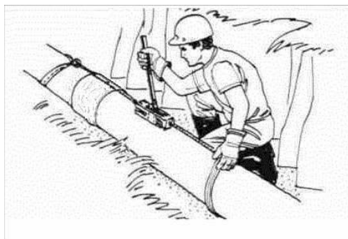
Рисунок Б.10 – Технологические операции монтажа труб «Перфокор» в качестве элемента дренажной системы
