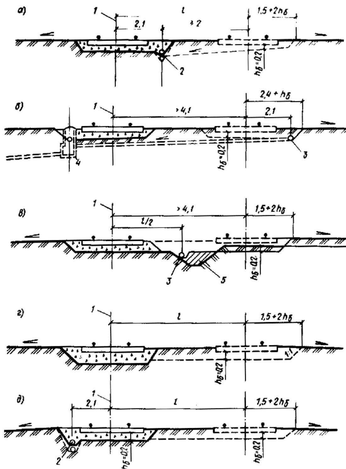
Рисунок В.42 – Схемы дорожного одностороннего дренажа
