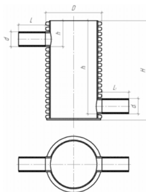
Рисунок Б.13 – Полиэтиленовый перепадной колодец
