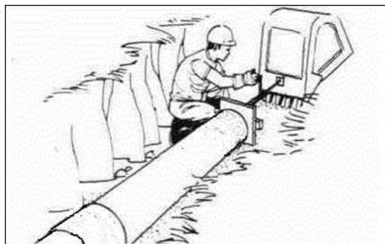
Рисунок Б.10 – Технологические операции монтажа труб «Перфокор» в качестве элемента дренажной системы
