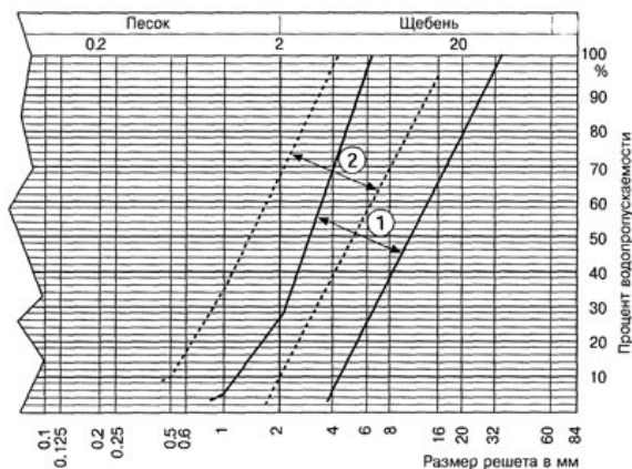
Рисунок В.32 – Водопрopusкная способность песка и щебня
