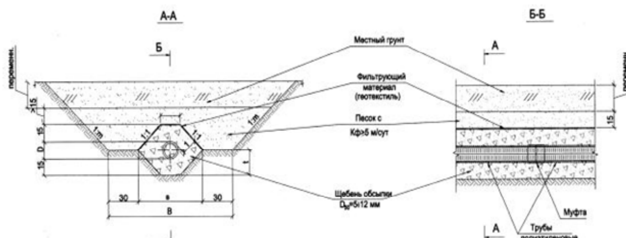
Рисунок В.23 – Вариант дренажа несовершенного типа в траншее с откосами шестиугольной формы и обсыпкой щебнем трубы «Перфокор»
