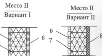
Рисунок В.53 – Поперечное сечение дрена с применением труб «Перфокор» и современных геосинтетических материалов
