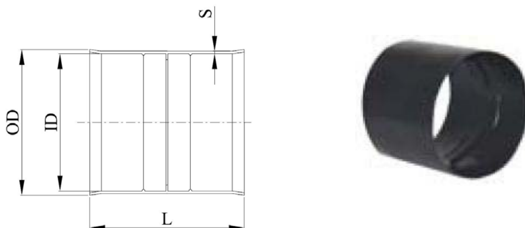
Рисунок Б.9 - Облегченная муфта для соединения труб «Перфокор» малого диаметра
