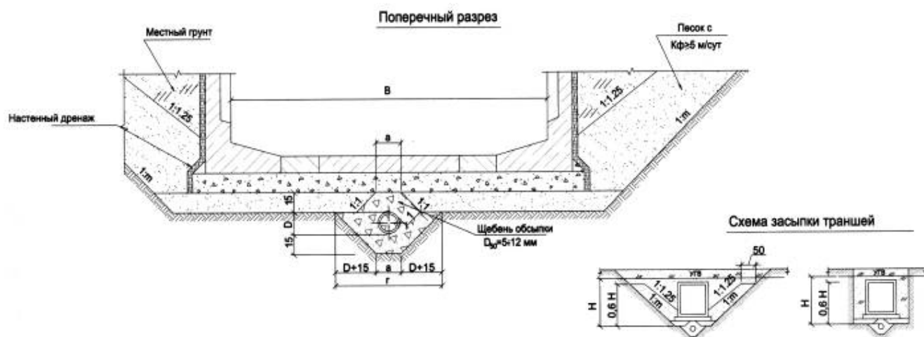
Рисунок В.30 – Вариант дренажа коллектора несовершенного типа трапециидальной формы с обсыпкой щебнем трубы «Перфокор»
