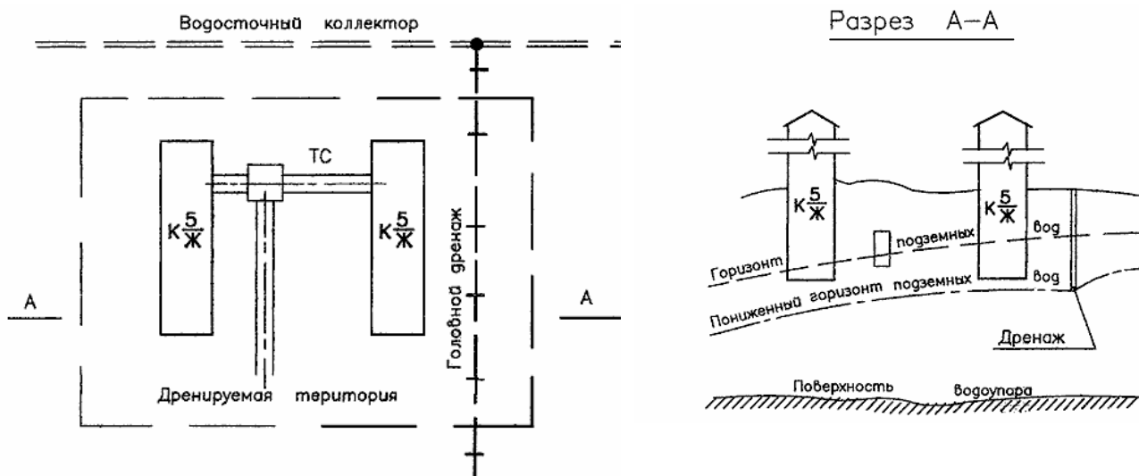
Рисунок В.4 – Головной траншейный дренаж
