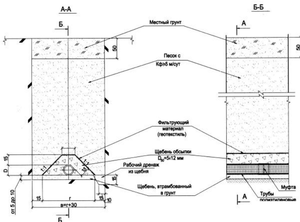
Рисунок В.25 – Вариант дренаж несовершенного типа трапециидальной формы с обсыпкой щебнем трубы «Перфоркор»
