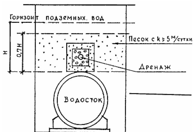
Рисунок В.38 – Прокладка дренажа над водосток с применением труб «Перфокор»
