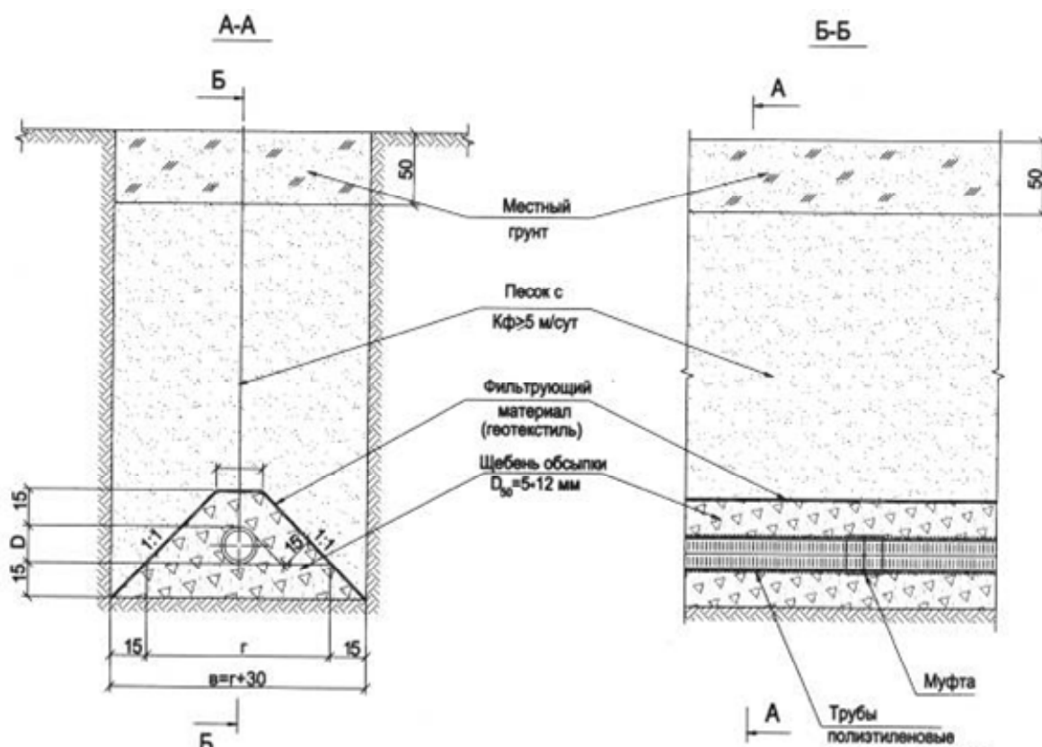
Рисунок В.20 – Вариант траншейго дренажа несовершенного типа трапециидальной формы с обсыпкой щебнем трубы «Перфокор»
