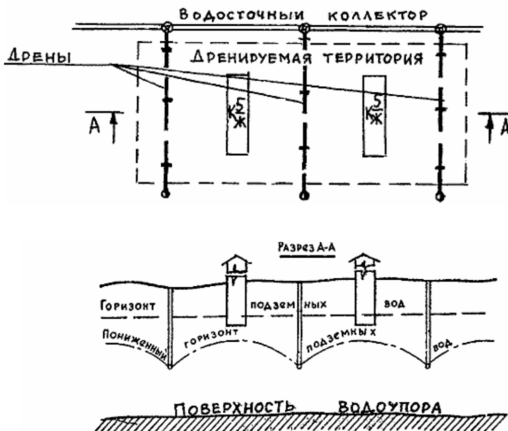
Рисунок В.5 – Систематический траншейный дренаж
