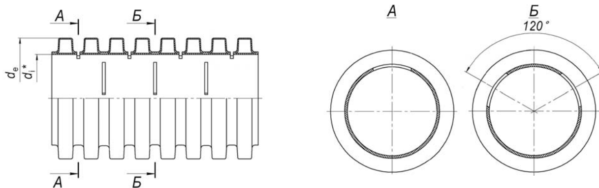
Рисунок Б.2 - Дренажная труба «Перфокор-П» для диаметров 110-160 мм. Частичное перфорирование
