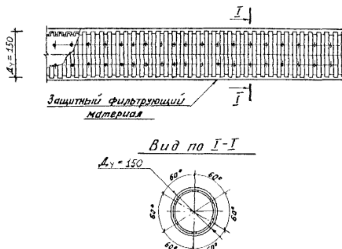
Рисунок В.33 – Оболочка – фильтр из геотекстиля на трубе «Перфокор»
