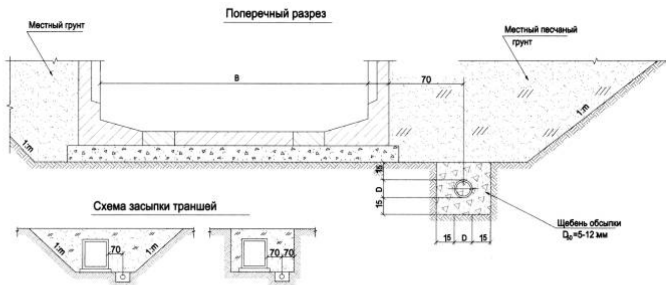
Рисунок В.31 – Вариант дренажа коллектора несовершенного типа прямоугольной формы с обсыпкой щебнем трубы «Перфокор»
