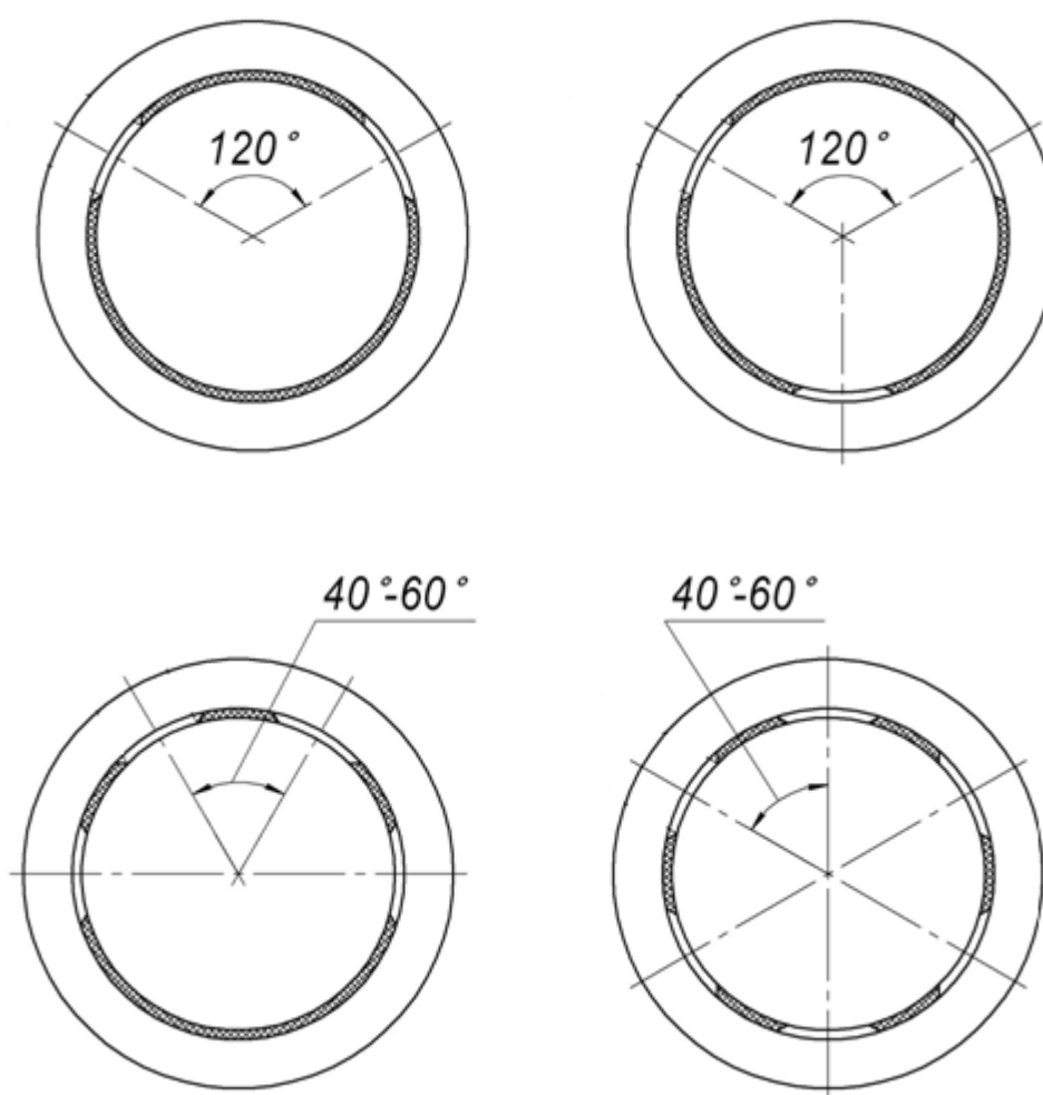
Рисунок Б.3— Дренажная труба «Перфокор-П» для диаметров 200-630 мм. Расположение водоприемных отверстий
