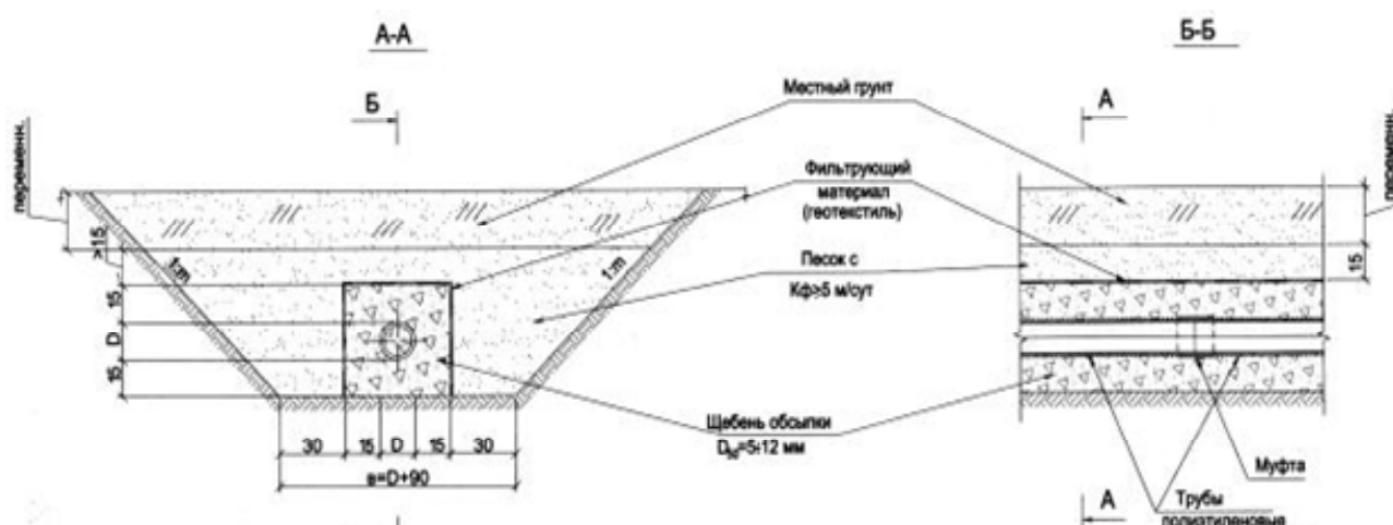
Рисунок В.21 – Вариант дренажа несовершенного типа в траншее с откосами прямоугольной формы и обсыпкой щебнем трубы «Перфокор»
