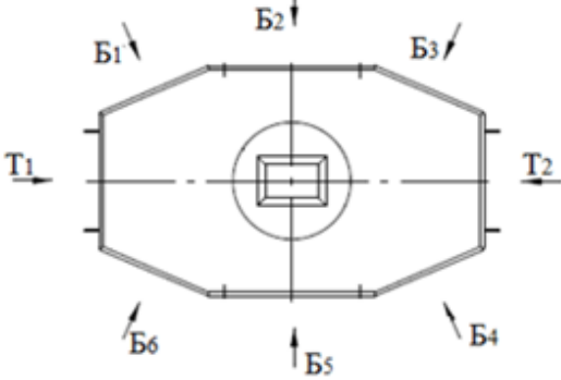
Схема обозначения сторон ККС-3,5-80 ССД-Пайп (вид сверху)
