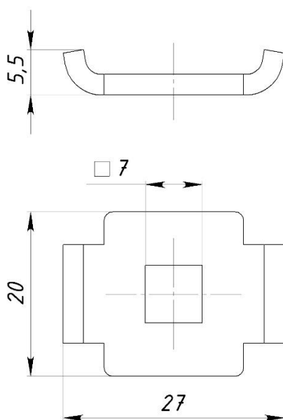
Рисунок 1 – Общий вид соединителя
