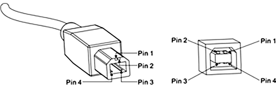
Figura 8. Porta USB
