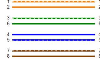
Схема разводки (T568B)
