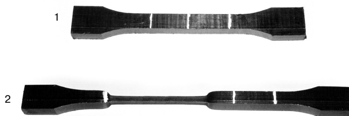
Фото 3.1. Испытание ПЭ трубы на осевое растяжение (относительное удлинение при разрыве) является одним из эффективных способов проверки качества труб при осуществлении входного контроля. В аттестованной лаборатории из отрезка ПЭ трубы изготавливают образец (1). Контроль качества на соответствие стандарту проходит путем механического испытания образца на разрывной машине. Изготовленная в соответствии с требованиями стандарта труба должна обеспечить в ходе испытаний (2) необходимую величину удлинения (не менее 350%) до разрыва в соответствии с ГОСТ 18599-2001, ГОСТ Р 50838-2009.
