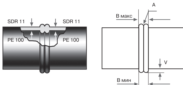
Рис. 4.2.19. Параметры грата
