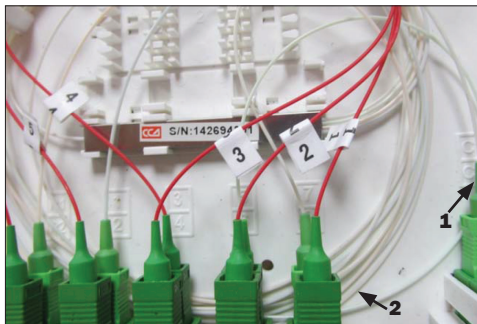
1 – оптический шнур входа разветвителя; 2 – оптические шнуры выходов разветвителя
