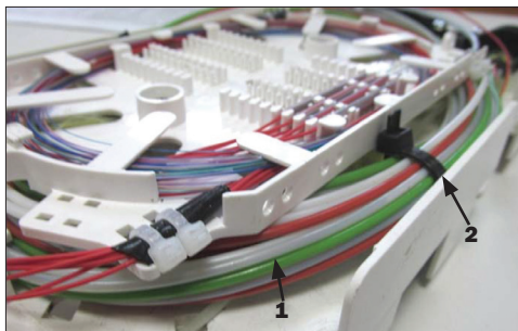
1 – уложенный запас длины «транзитных» ОМ; 2 – одно из мест фиксации «транзитных» ОМ
