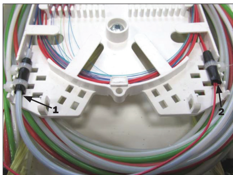
1 – ответвляемый ОМ; 2 – шнур «пигтейл» для подключения ОВ кабеля направления «А» к входу разветвителя
