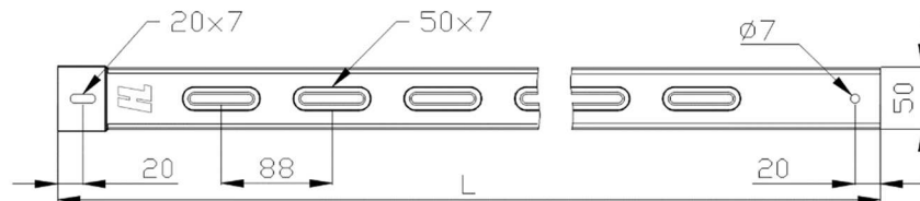
Рисунок 2 – Параметр перфорации лотка с шириной лотка 50 мм
