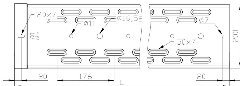
Рисунок 5 – Параметр перфорации лотка с шириной лотка 200 мм
