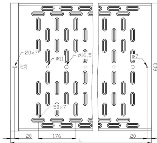
Рисунок 9 – Параметр перфорации лотка с шириной лотка 600 мм
