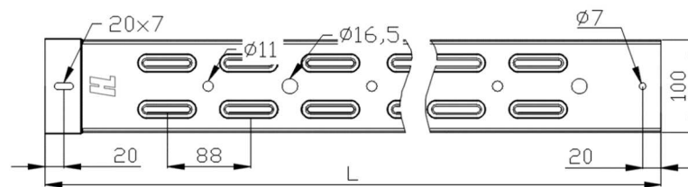
Рисунок 3 – Параметр перфорации лотка с шириной лотка 50 мм
