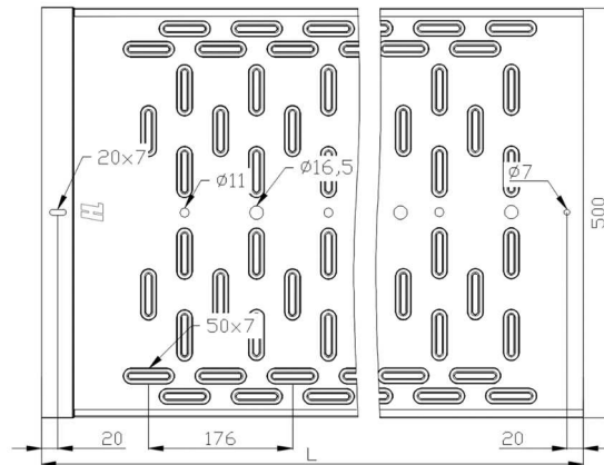
Рисунок 8 – Параметр перфорации лотка с шириной лотка 500 мм
