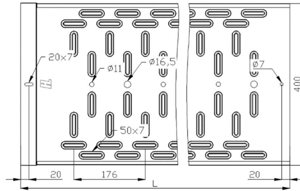
Рисунок 7 – Параметр перфорации лотка с шириной лотка 400 мм
