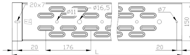
Рисунок 4 – Параметр перфорации лотка с шириной лотка 150 мм
