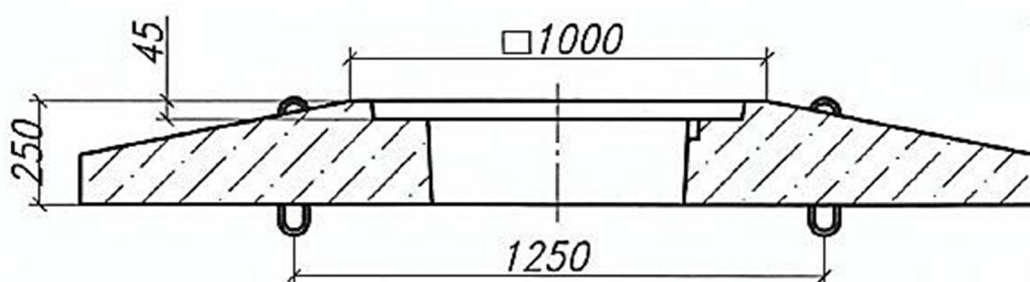
Рис. 4. Размеры плиты ОП-1-У, продольный разрез.
