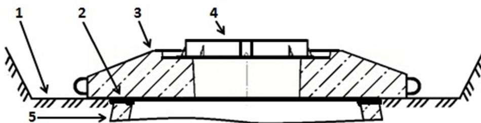
Рис. 11. Плита ОП-1-У установлена на колодец с удалённым перекрытием.
