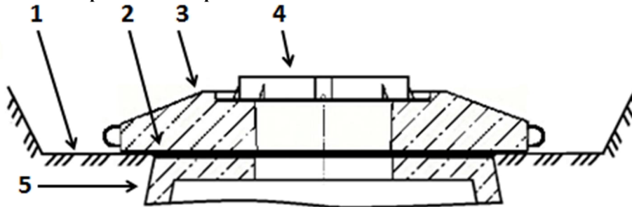
Рис. 7. Плита ОП-1-У установлена на перекрытие колодца при новом строительстве.
