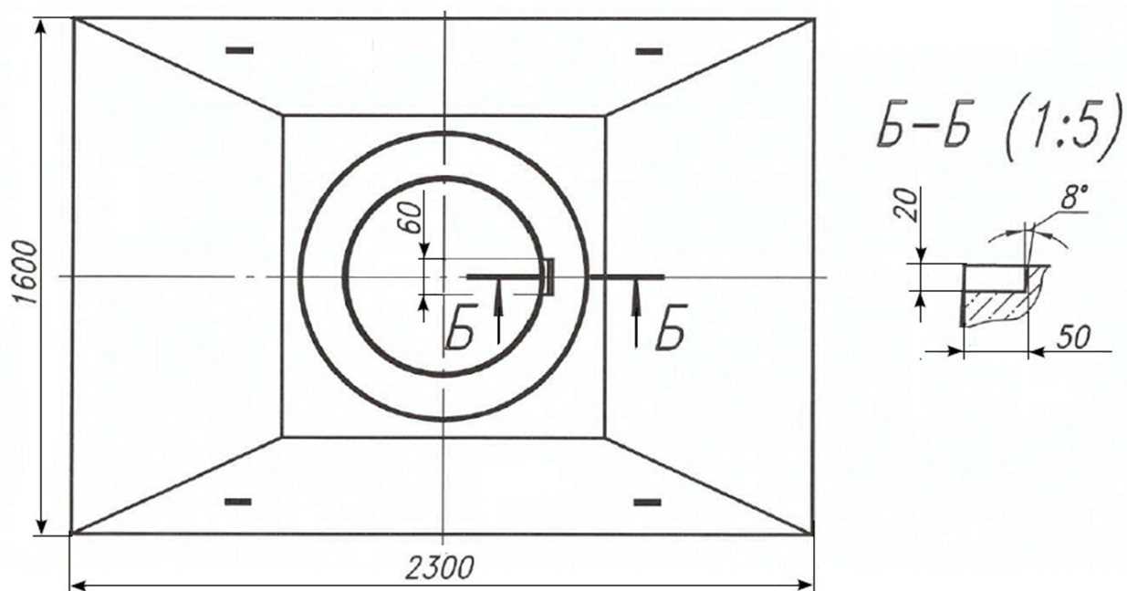
Рис. 3. Размеры плиты ОП-1-У, вид сверху.
