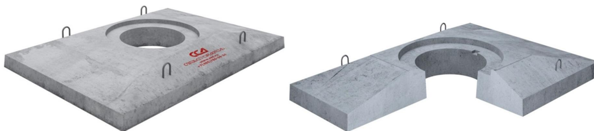
Рис. 1. Разгрузочная плита ОП-1-У: внешний вид и разрез.
