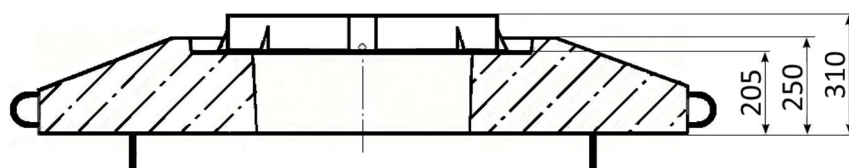
Рис. 8. Высота плиты с люком при установке его непосредственно в плиту.
