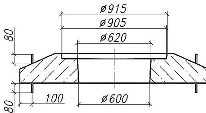
Рис. 5. Размеры плиты ОП-1-У, поперечный разрез.
