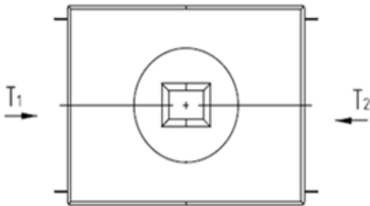
Схема обозначения сторон ККС-2,5-80 ССД-Пайп (вид сверху)
