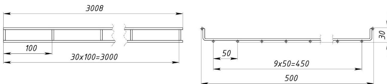
Рисунок 8 – Конструктивное исполнение лотков с шириной 500 мм и высотой 30 мм
