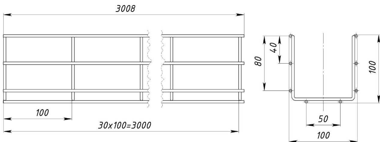
Рисунок 24 – Конструктивное исполнение лотков с шириной 100 мм и высотой 100 мм
