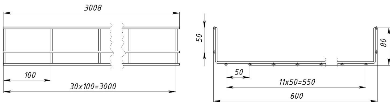
Рисунок 23 – Конструктивное исполнение лотков с шириной 600 мм и высотой 80 мм
