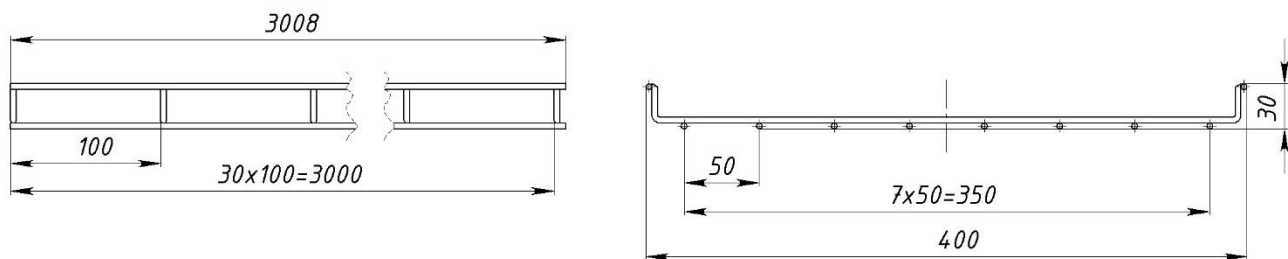
Рисунок 7 – Конструктивное исполнение лотков с шириной 400 мм и высотой 30 мм
