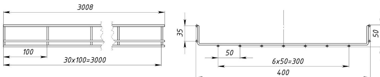
Рисунок 14 – Конструктивное исполнение лотков с шириной 400 мм и высотой 50 мм
