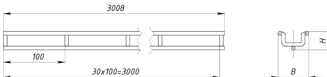
Рисунок 2 – Конструктивное исполнение лотков с шириной 50 и 60 мм
