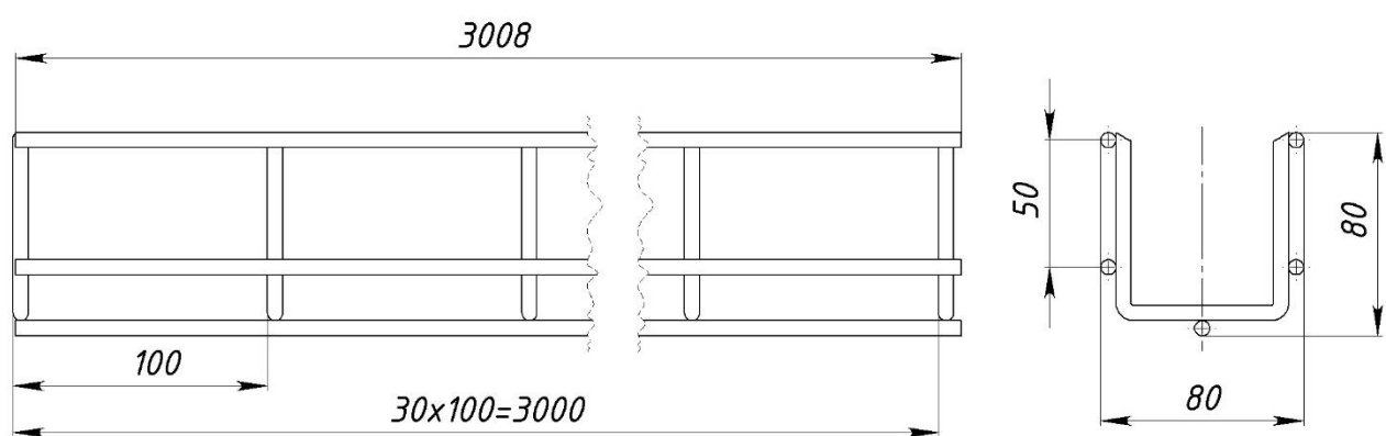
Рисунок 31 – Конструктивное исполнение лотков с шириной 80 мм и высотой 80 мм
