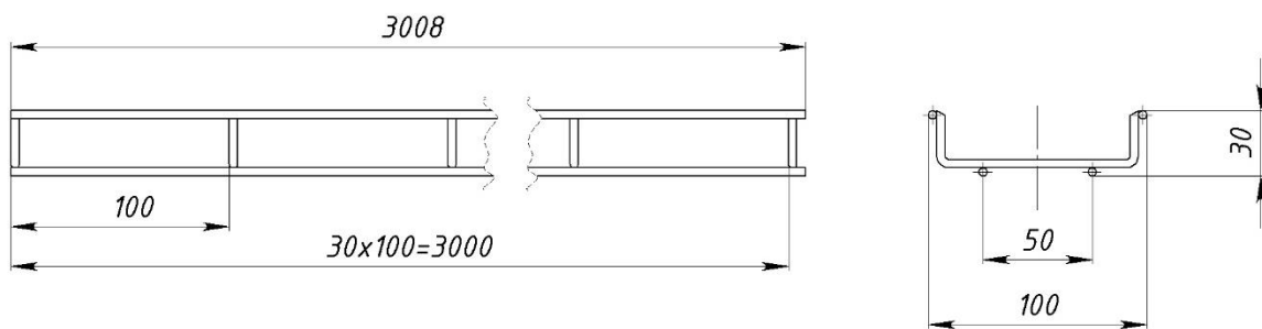
Рисунок 3 – Конструктивное исполнение лотков с шириной 100 мм и высотой 30 мм
