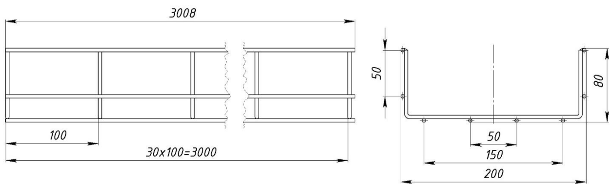
Рисунок 19 – Конструктивное исполнение лотков с шириной 200 мм и высотой 80 мм
