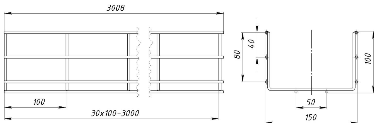
Рисунок 25 – Конструктивное исполнение лотков с шириной 150 мм и высотой 100 мм
