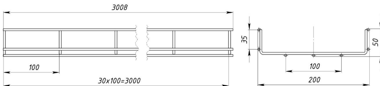
Рисунок 12 – Конструктивное исполнение лотков с шириной 200 мм и высотой 50 мм
