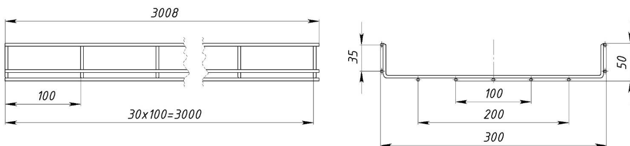
Рисунок 13 – Конструктивное исполнение лотков с шириной 300 мм и высотой 50 мм
