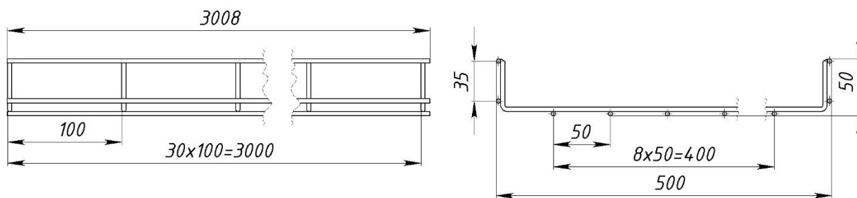
Рисунок 15 – Конструктивное исполнение лотков с шириной 500 мм и высотой 50 мм
