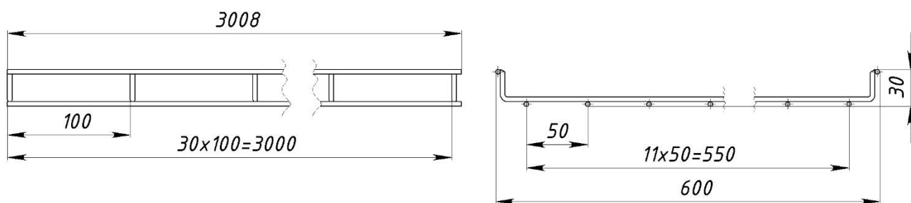
Рисунок 9 – Конструктивное исполнение лотков с шириной 600 мм и высотой 30 мм
