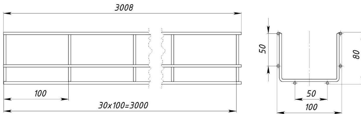
Рисунок 17 – Конструктивное исполнение лотков с шириной 100 мм и высотой 80 мм
