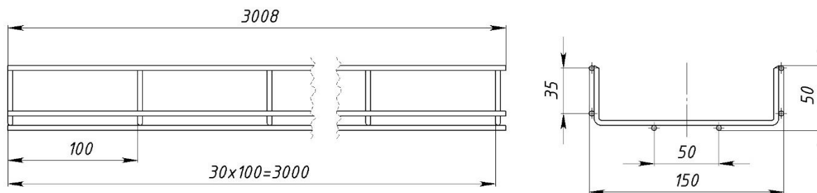
Рисунок 11 – Конструктивное исполнение лотков с шириной 150 мм и высотой 50 мм
