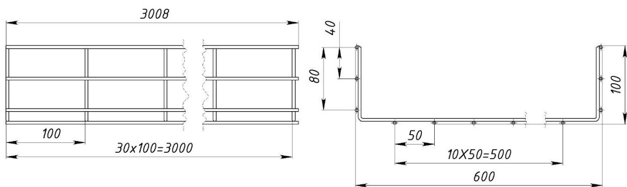
Рисунок 30 – Конструктивное исполнение лотков с шириной 600 мм и высотой 100 мм
