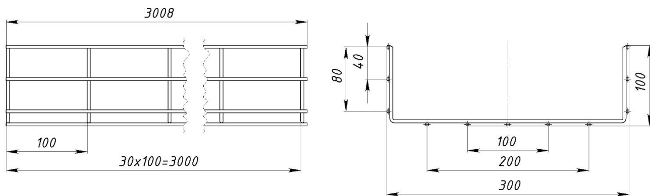
Рисунок 27 – Конструктивное исполнение лотков с шириной 300 мм и высотой 100 мм
