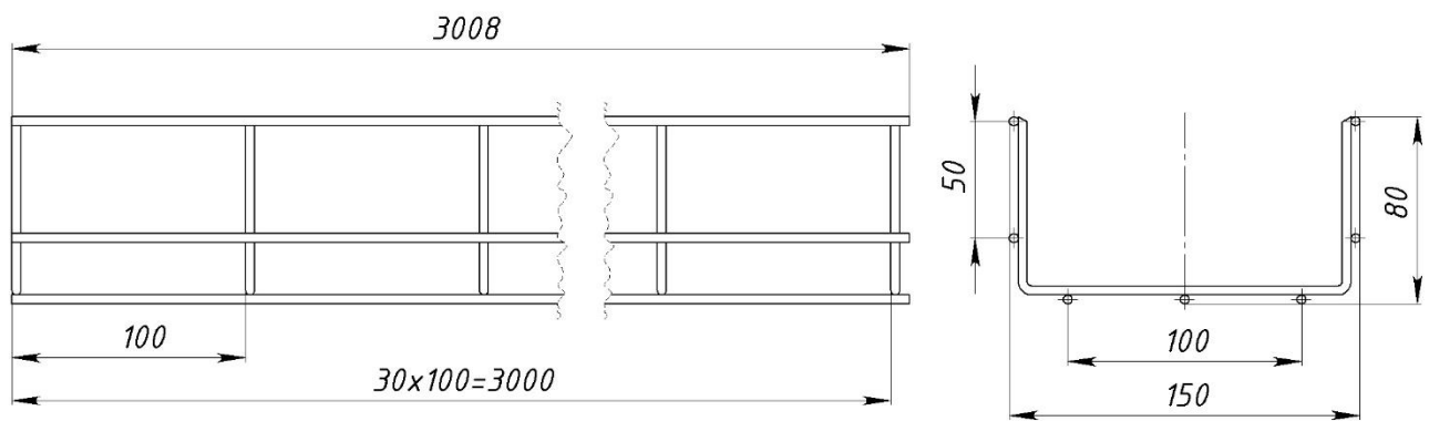
Рисунок 18 – Конструктивное исполнение лотков с шириной 150 мм и высотой 80 мм
