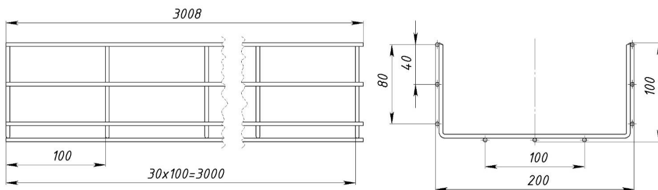
Рисунок 26 – Конструктивное исполнение лотков с шириной 200 мм и высотой 100 мм
