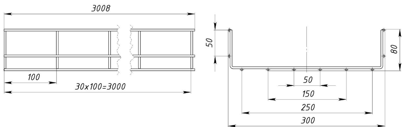
Рисунок 20 – Конструктивное исполнение лотков с шириной 300 мм и высотой 80 мм
