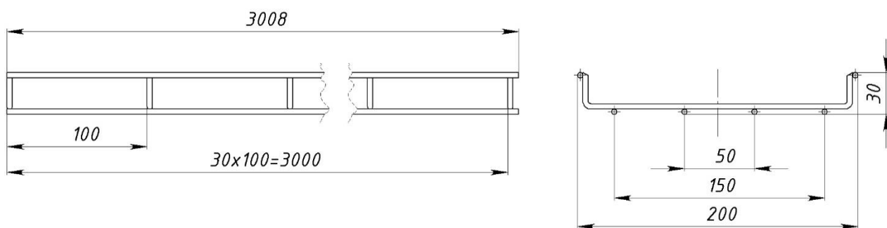
Рисунок 5 – Конструктивное исполнение лотков с шириной 200 мм и высотой 30 мм
