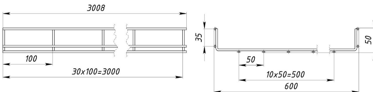
Рисунок 16 – Конструктивное исполнение лотков с шириной 600 мм и высотой 50 мм
