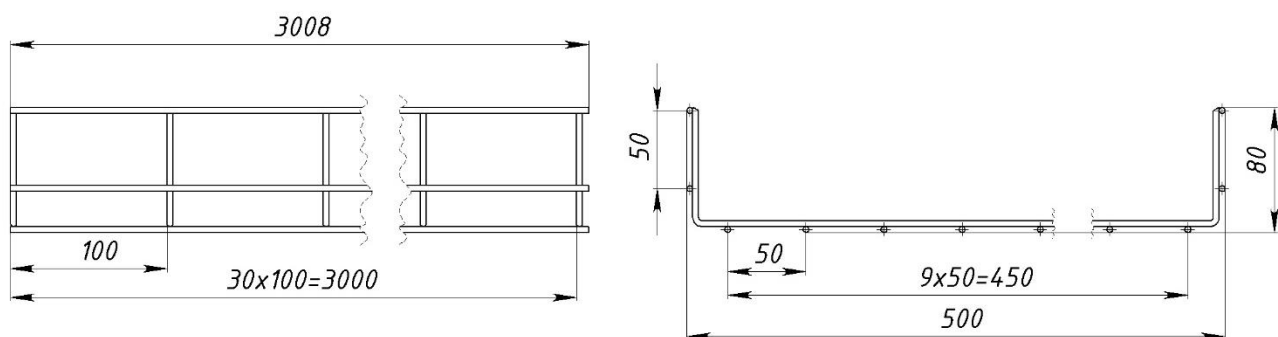
Рисунок 22 – Конструктивное исполнение лотков с шириной 500 мм и высотой 80 мм
