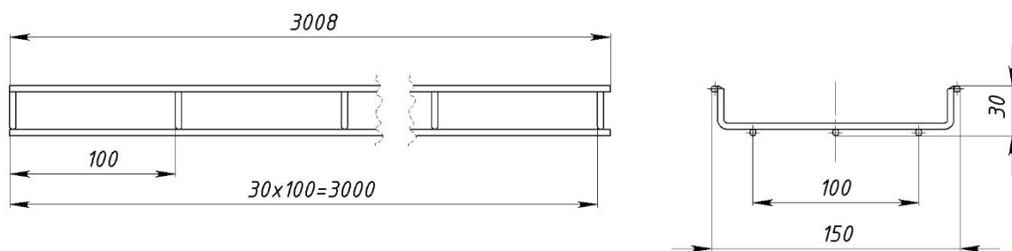
Рисунок 4 – Конструктивное исполнение лотков с шириной 150 мм и высотой 30 мм
