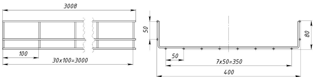
Рисунок 21 – Конструктивное исполнение лотков с шириной 400 мм и высотой 80 мм
