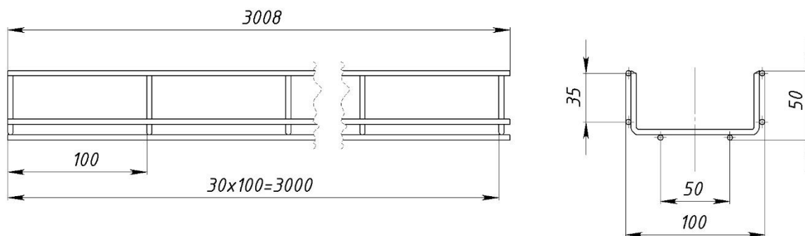
Рисунок 10 – Конструктивное исполнение лотков с шириной 100 мм и высотой 50 мм
