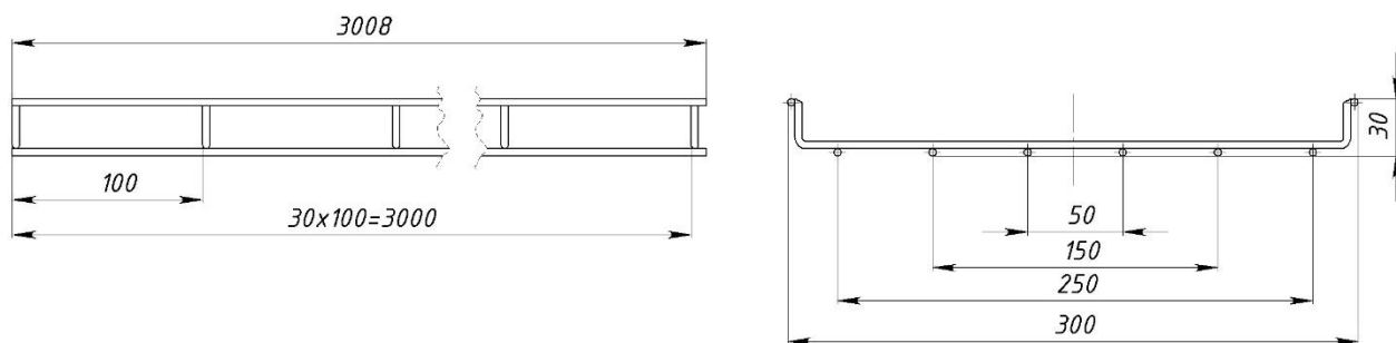
Рисунок 6 – Конструктивное исполнение лотков с шириной 300 мм и высотой 30 мм
