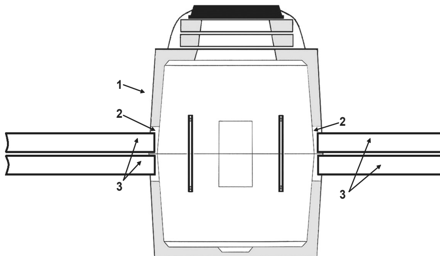
Рис. 9. Ввод труб в колодец «ККСр-2-10(80)»: 1 – торцевая стена колодца; 2 – проёмы в торцевых стенках; 3 – хризотилцементные (асбестоцементные) трубы.
