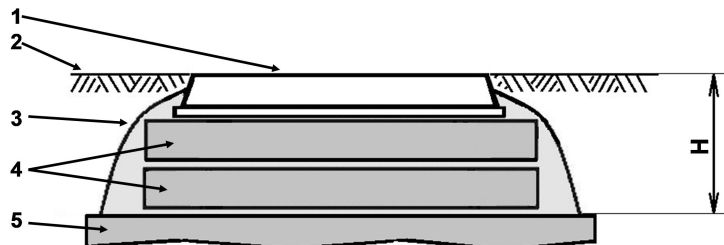
Рис. 11. Расстояние от перекрытия колодца до уровня земли (асфальта) – H:
