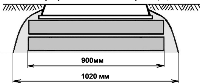
Рис. 12. Размеры (диаметры) опорных колец типа КО и бетонной обмазки.
