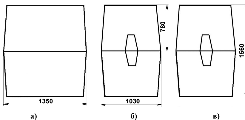
Рис. 6. Габаритные размеры колодца «ККСр-2-10(80)»: а - вид сбоку; б и в – вид с торца.
