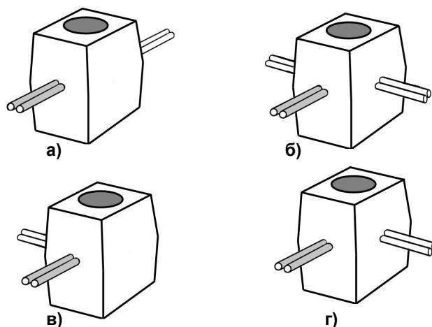
Рис. 3. Варианты использования колодца «ККСр-2-10(80)».
