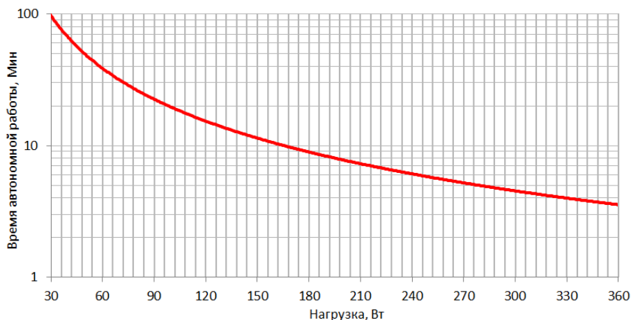
Рисунок 5. График автономной работы INFO600 / INFOLCD600
