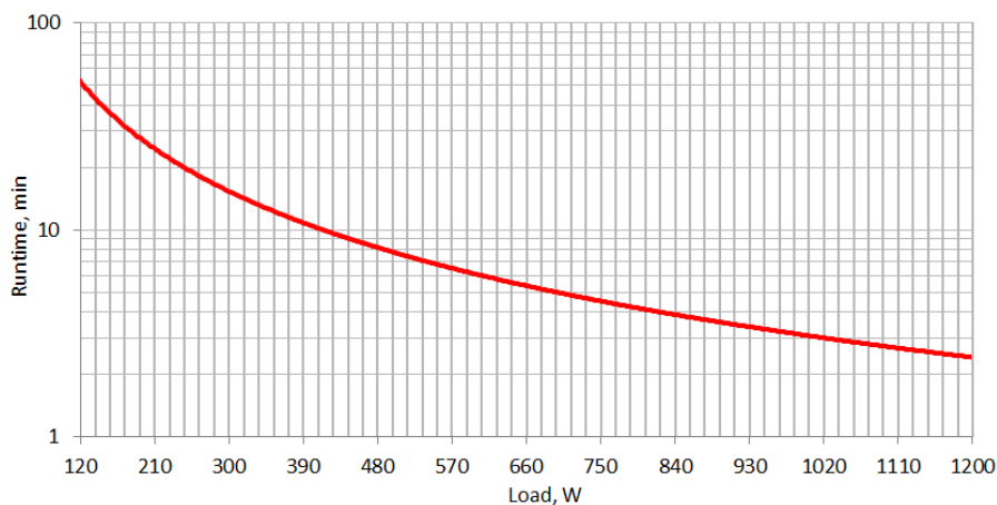
Figure 7. Grafico durata batterie INFO2000 / INFOLCD2000
