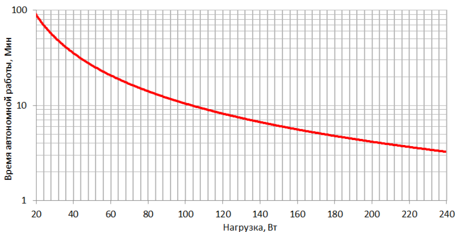
Рисунок 4. График автономной работы INFO400 / INFOLCD400
