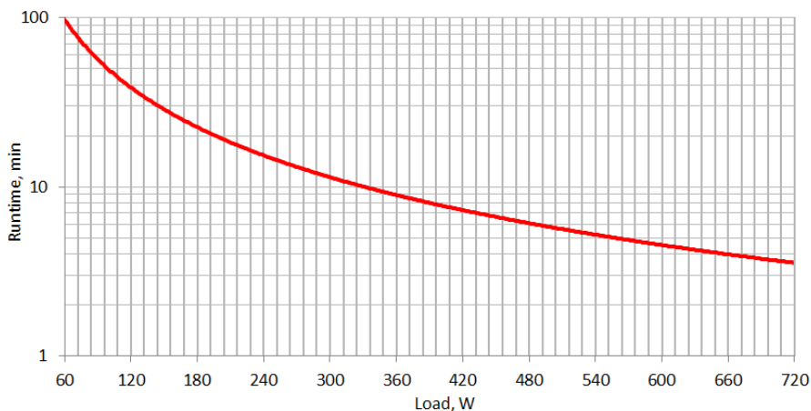
Figure 5. Grafico durata batterie INFO1200 / INFOLCD1200
