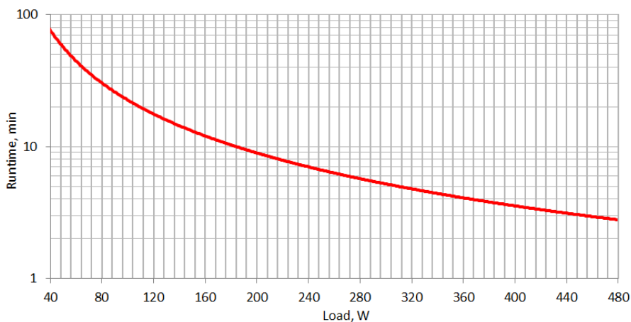
Figure 4. Grafico durata batterie INFO800 / INFOLCD800
