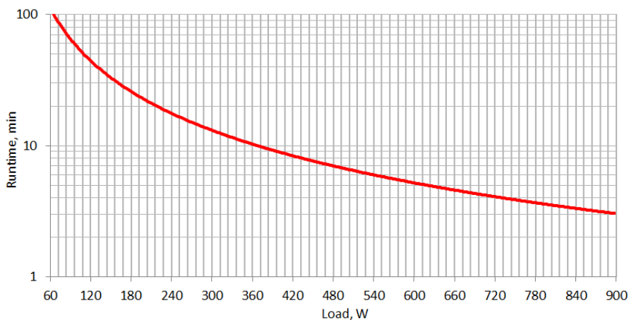
Figure 6. Grafico durata batterie INFO1500 / INFOLCD1500
