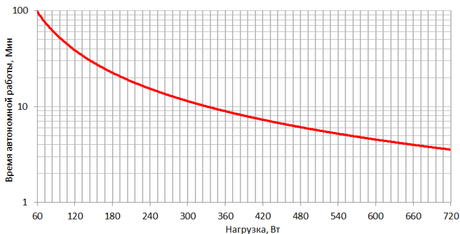
Рисунок 7. График автономной работы INFO1200 / INFOLCD1200
