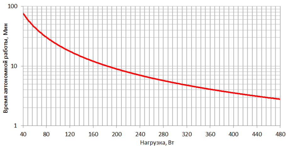
Рисунок 6. График автономной работы INFO800 / INFOLCD800
