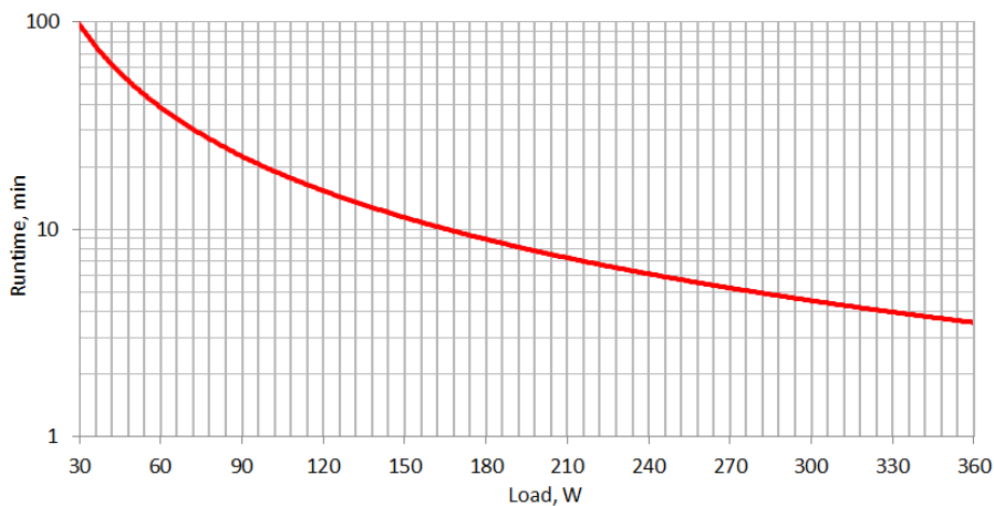
Figure 3. Grafico durata batterie INFO600 / INFOLCD600
