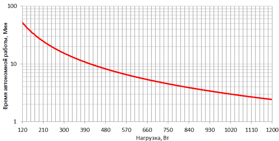
Рисунок 9. График автономной работы INFO2000 / INFOLCD2000
