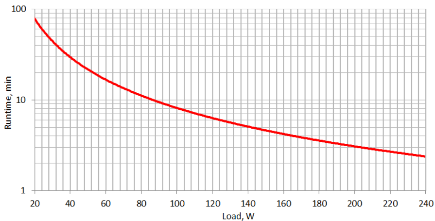
Figure 2. Grafico durata batterie INFO400 / INFOLCD400
