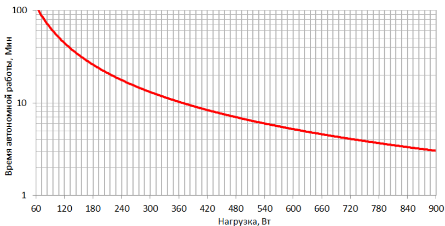
Рисунок 8. График автономной работы INFO1500 / INFOLCD1500
