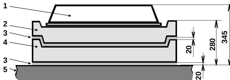
Рис. 14. Высота горловины с парой колец «КО-ЧП» и «КО-Ч»: 1 – люк чугунный типа «Т»; 2 – кольцо «КО-Ч»; 3 – слой бетона со щебнем; 4 – кольцо «КО-ЧП»; 5 – перекрытие колодца «ККСр-5-80».
