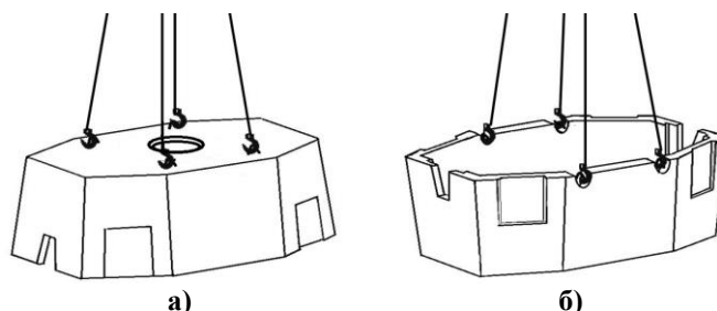
Рис. 9. Строповка элементов «ККСр-5-80»: а – верхнего элемента; б – нижнего элемента.
