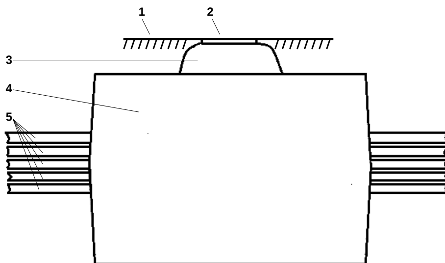
Рис. 2. Колодец «ККСр-5-80» как подземное сооружение: 1 – уровень земли или асфальта; 2 – чугунный люк; 3 – горловина в бетонной обмазке; 4 – корпус колодца в сборе; 5 – вводимые каналы, 24 трубы.
