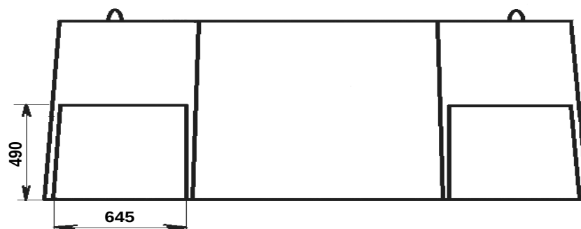
Рис. 7. Размеры ниши на примере верхнего элемента колодца «ККСр-5-80». На нижнем элементе ниши такого же размера.
