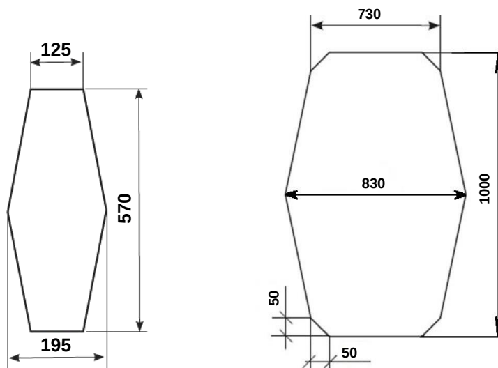
Рис. 2.2. Размеры технологического отверстия и участка с тонкой неармированной стенкой на торцевой стене колодца «ККСр-5-80».
