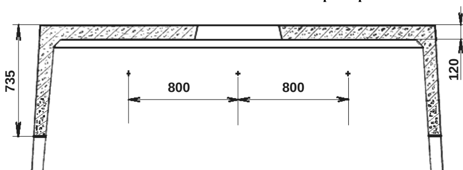
Рис. 7. Размеры ниши на примере верхнего элемента колодца «ККСр-5-80». На нижнем элементе ниши такого же размера.
