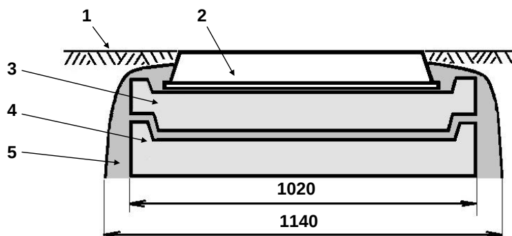
Рис. 15 Диаметры колец и обсаженной бетоном горловины при использовании пары «КО-ЧП» и «КО-Ч»: 1 – уровень дорожного покрытия; 2 – люк тяжёлого типа; 3 – кольцо «КО-Ч»; 4 – кольцо «КО-ЧП»; 5 - обсадка горловины бетоном со щебнем.
