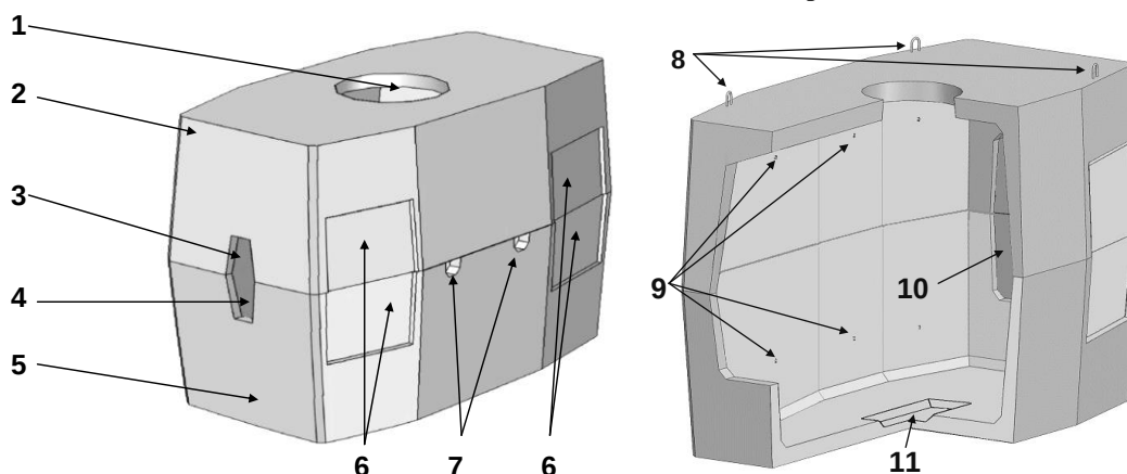
Рис. 4. Колодец «ККСр-5-80», внешний вид и детали элементов колодца: 1 – круглое отверстие для люка; 2 – верхний элемент; 3 – технологическое отверстие верхнего элемента; 4 – технологическое отверстие нижнего элемента; 5 – нижний элемент; 6 – ниши на наружных поверхностях боковых стен; 7 – гнезда с подъёмными петлями на нижнем элементе; 8 – подъёмные петли на перекрытии; 9 – отверстия для ершей; 10 – участки с тонкими неармированными стенками вокруг технологических отверстий в элементах; 11 – приямок для стока воды.
