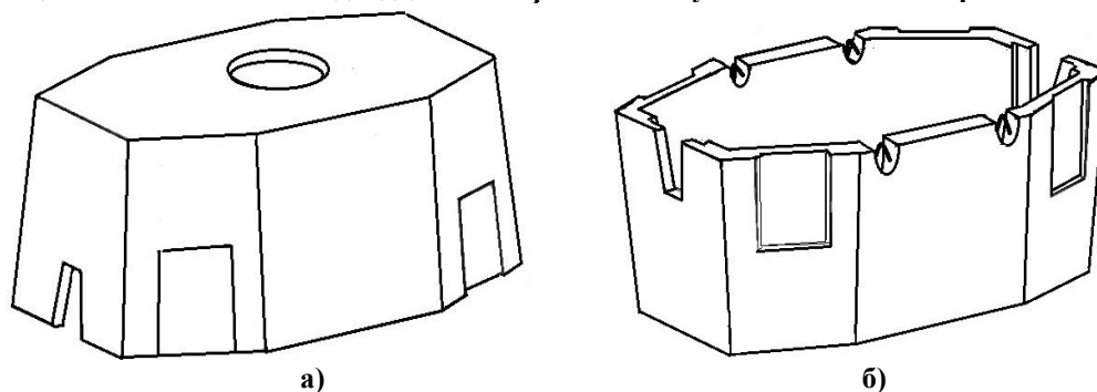
Рис. 1. Колодец «ККСр-5-80» как изделие: а – верхний элемент колодца; б – нижний элемент.
