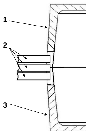
Рис. 11. Ввод труб в колодец «ККСр-5-80»: 1 – торцевая стена верхнего элемента колодца; 2 – ввод хризотилцементных труб в проёмы в торцевых стенах элементов колодца; 3 – торцевая стена нижнего элемента колодца.
