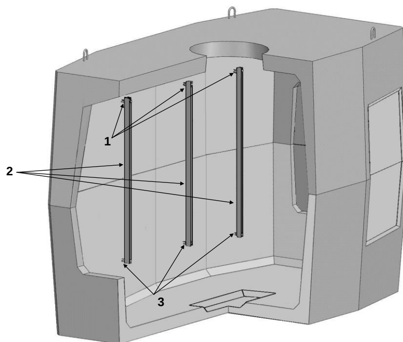
Рис. 3.1. Кронштейны «ККП-130» на боковой стене колодца «ККСр-5-80»: 1 – ерши в верхнем элементе; 2 - кронштейны; 3 – ерши в нижнем элементе.
