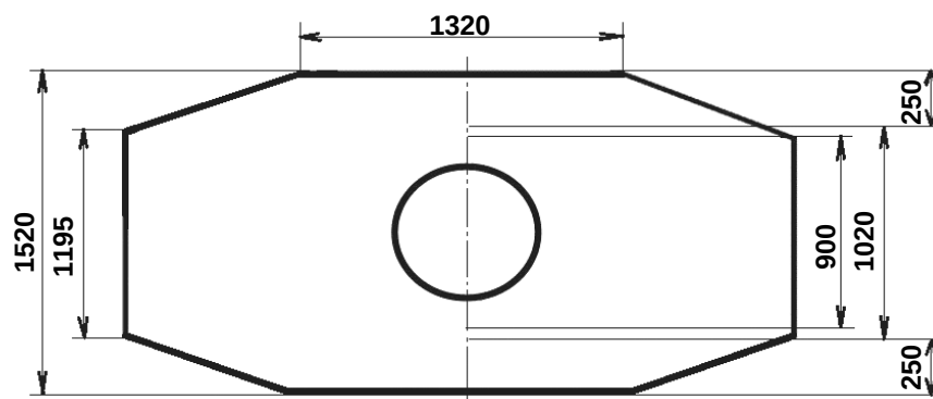
Рис. 6. Размеры перекрытия колодца «ККСр-5-80» с указанием диаметров опорных колец: 900 мм – кольца типа КО; 1020 мм – кольца КО-ЧП и КО-Ч.
