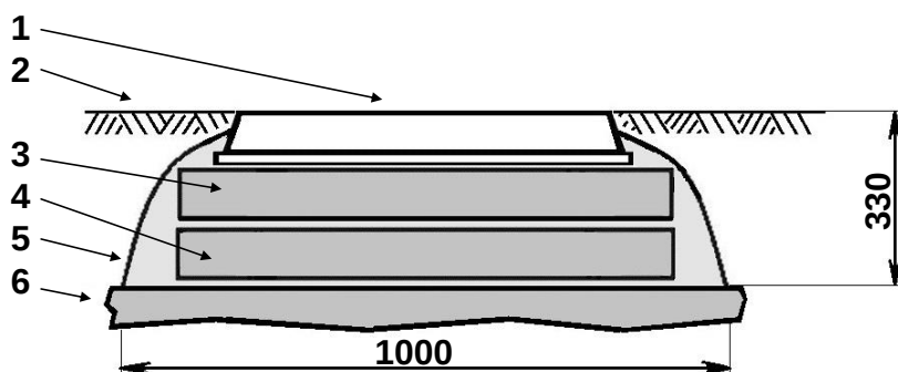
Рис. 13. Горловина с кольцами типа КО и люком типа «Т»:
