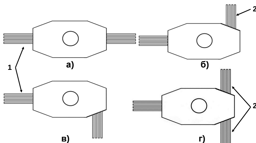
Рис. 3. Классический примеры использования колодца «ККСр-5-80»*: 1 – вводимые каналы; 2 – ответвляющиеся каналы; а - проходной колодец; б, в – угловые колодцы; г - разветвительный колодец.
