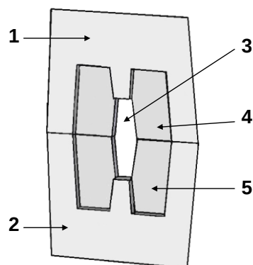
Рис. 2.1. Участок с тонкой неармированной стенкой на торцевой стене колодца «ККСр-5-80»:
