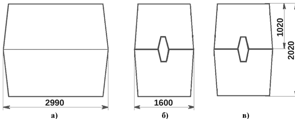
Рис. 5. Габаритные размеры колодца «ККСр-5-80»:
