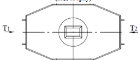
Схема обозначения сторон ККС-4-10 ССД-Пайп (вид сверху)
