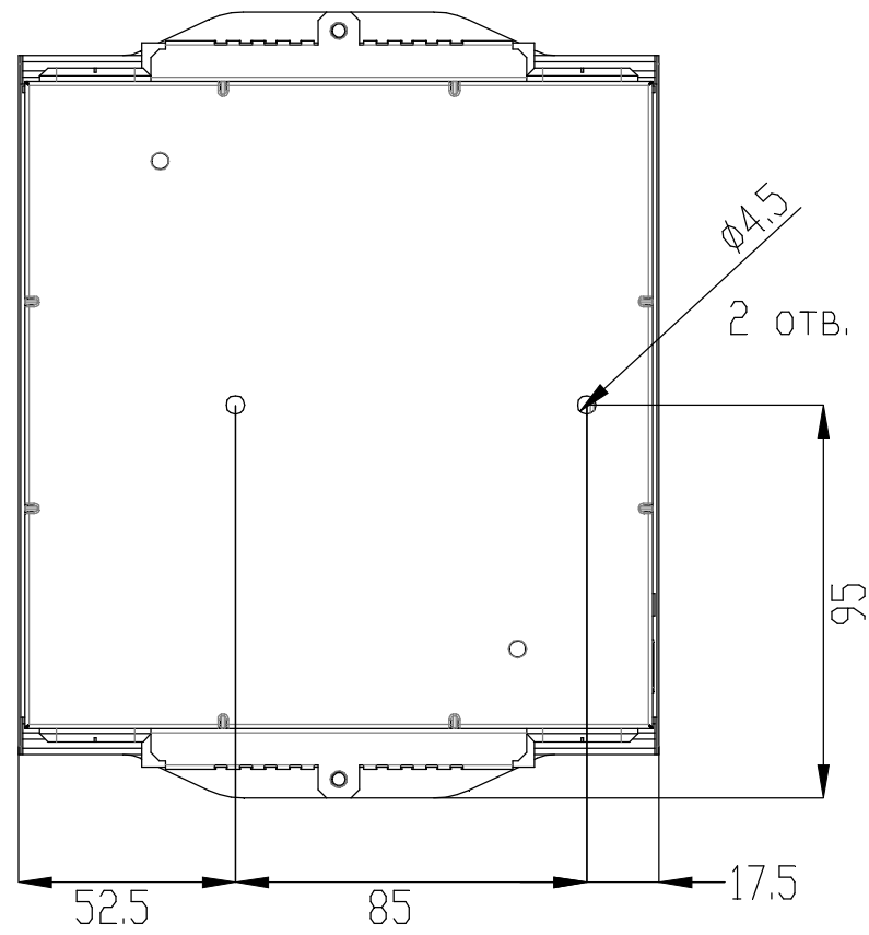
Расположение крепежных отверстий
