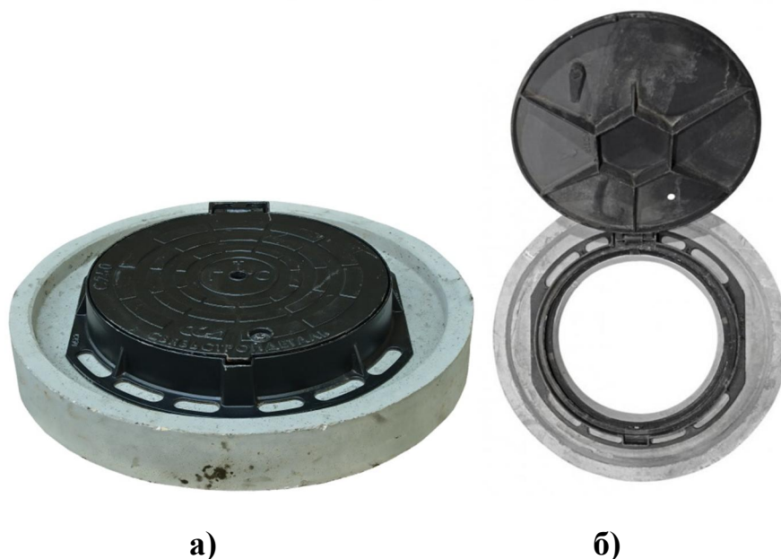
Рис. 10. Люк из ВЧШГ ГТС тяжёлого типа установлен на кольцо КО-Ч: а – чугунная крышка закрыта; б – чугунная крышка открыта.
