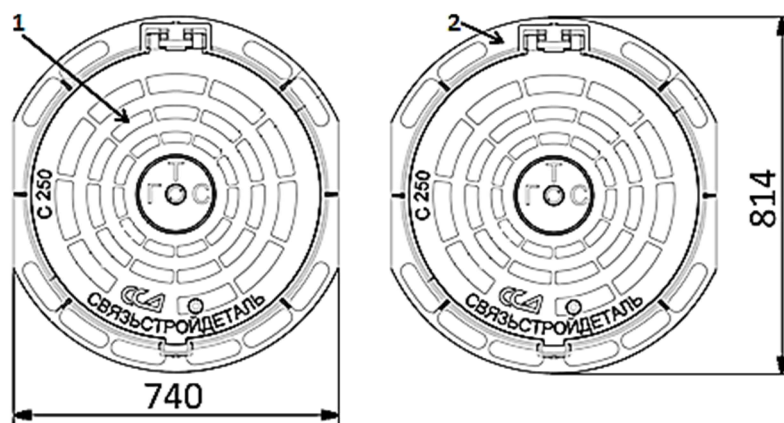
Рис. 9. Детали и размеры люка из ВЧШГ ГТС тяжёлого типа: 1 – верхняя крышка; 2 – корпус.
