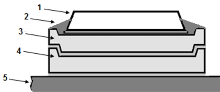
Рис. 6. Обмазка люка на горловине из колец КО-ЧП и КО-Ч: 1 – люк чугунный тяжёлого типа; 2 – обмазка из бетона со щебнем до середины высоты люка; 3 – кольцо «КО-Ч»; 4 – кольцо «КО-ЧП»; 5 – перекрытие колодца ККСр или ККСС.
