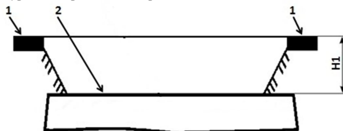
Рис. 7. Определение общей высоты горловины при ремонте: 1 – уровень дорожного покрытия и крышки чугунного люка; 2 – уровень перекрытия колодца; H1 – высота горловины от перекрытия колодца до уровня дорожного покрытия.
