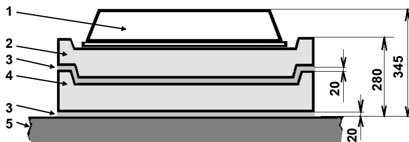
Рис. 5. Высота горловины с парой колец «КО-ЧП» и «КО-Ч»: 1 – люк чугунный типа «Т»; 2 – кольцо «КО-Ч»; 3 – слой бетона со щебнем; 4 – кольцо «КО-ЧП»; 5 – перекрытие колодца ККСр или ККСС.
