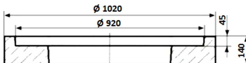
Рис. 2. Размеры опорного кольца КО-ЧП.
