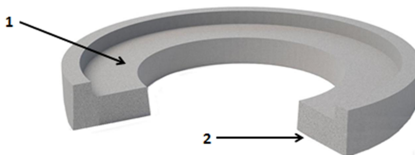
Рис. 1. Разрез кольца КО-ЧП, поясняющий особенности его конструкции: 1 – посадочное место для кольца КО-Ч; 2 – нижняя плоская поверхность.
