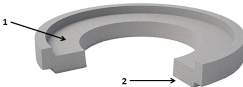
Рис. 3. Разрез кольца КО-Ч, поясняющий особенности его конструкции: 1 – посадочное место для люка; 2 – выступ (четверть) на нижней поверхности..
