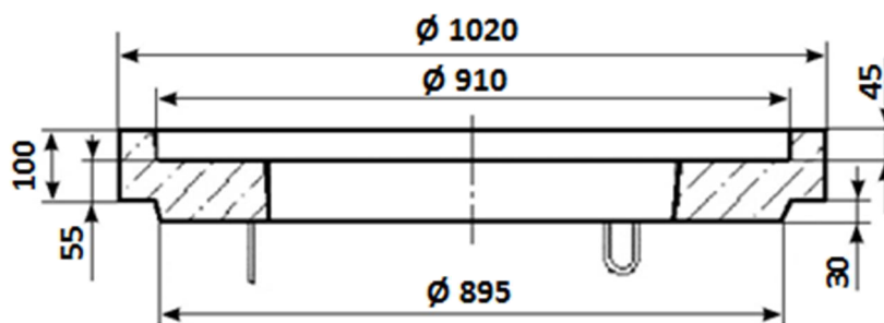
Рис. 4. Размеры опорного кольца КО-Ч.
